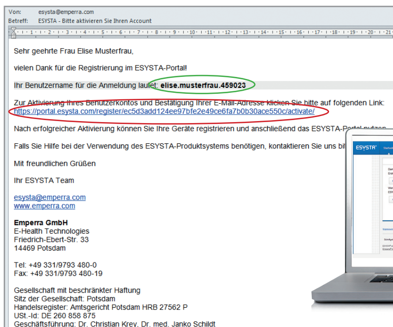
Muster Bestätigungs-E-Mail
